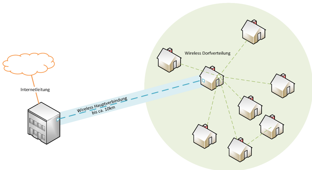
Schematische Darstellung einer Anbindung eines Weilers
